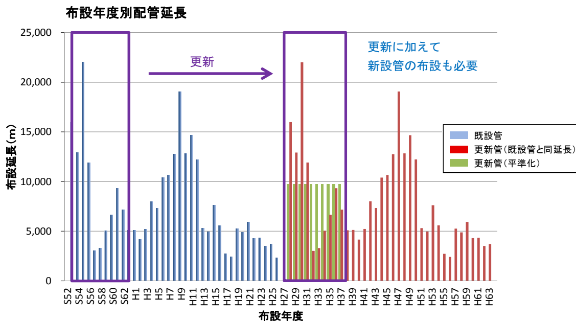
図 2.7 布設年度別配管延長と更新延長
